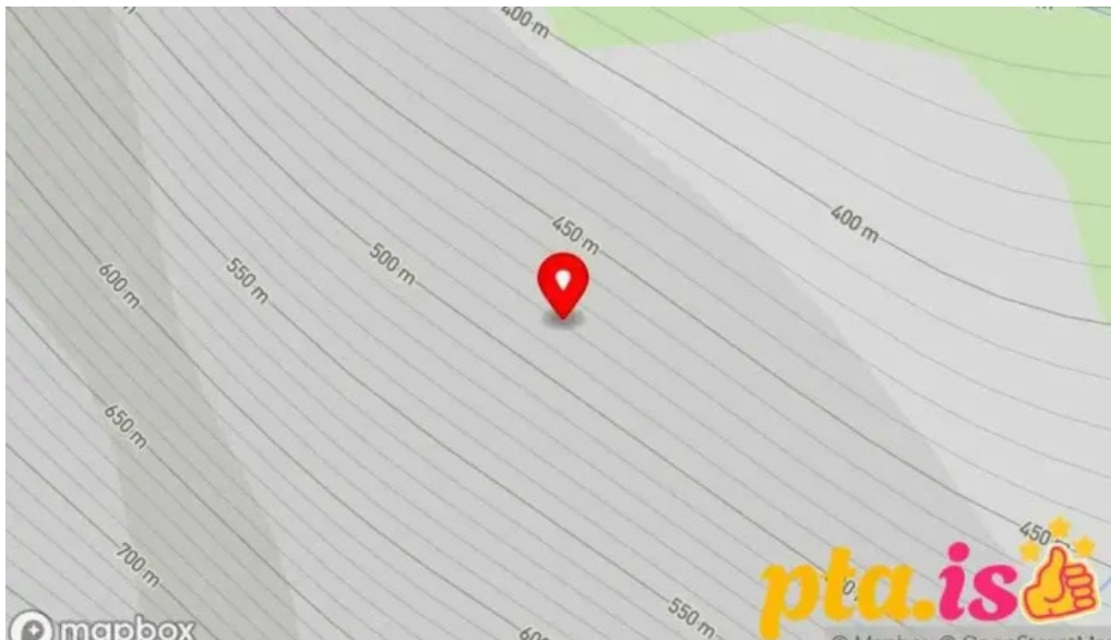
Breiðdalsvulkan iceland
